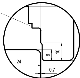
VARIANTE SENZA GUARNIZIONE
