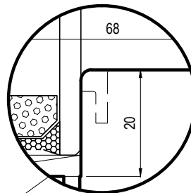
VARIANTE SENZA GUARNIZIONE
