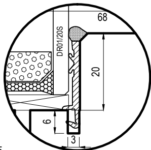
VARIANTE GUARNIZIONE ANTA
