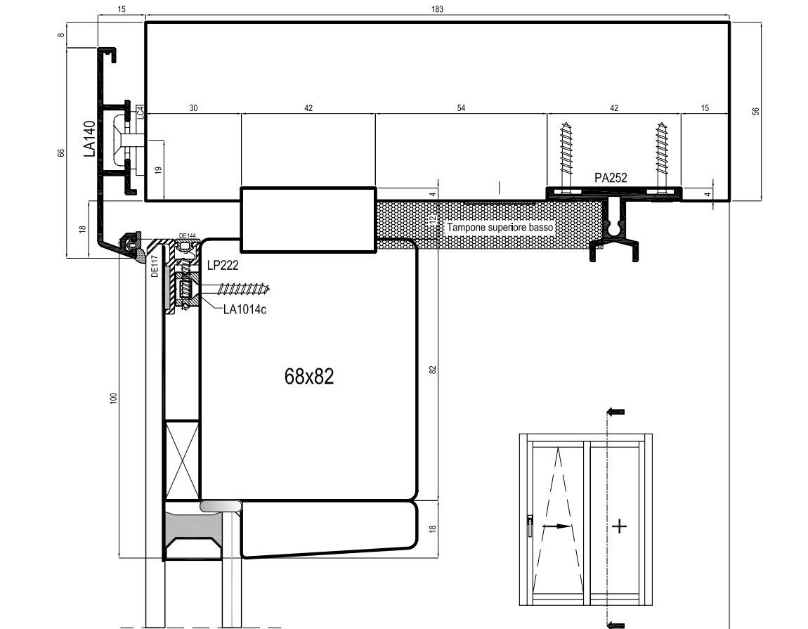
Sez. A-A
